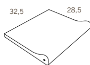
A BORDE PISCINA 28,5 28,5x32,5 cm · 11.2"x12.8"
