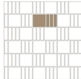
15 PIECES M 2 24,5x24,5 cm - 9.6"x9.6" 12 6x24,5 cm - 2.4"x9.6" 28 32,5x32,5 cm - 12.8"x12.8" 8 8x32,5 cm - 3.1"x12.8" 20
