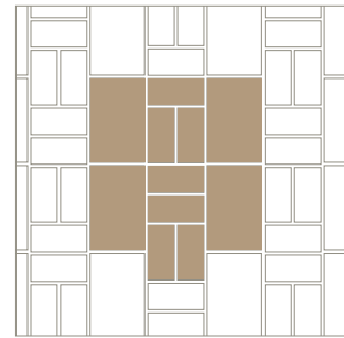
9 PIECES M 2 32,5x49,7 cm - 12.8"x19.6" 4 16x32,5 cm - 6.3"x12.8" 6
