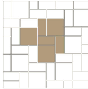
8 PIECES M 2 32,5x32,5 cm - 12.8"x12.8" 6,2 16x32,5 cm - 6.3"x12.8" 6,2
