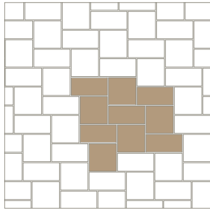
7 PIECES M 2 24,5x24,5 cm - 9.6"x9.6" 8,9 16x32,5 cm - 6.3"x12.8" 7,8
