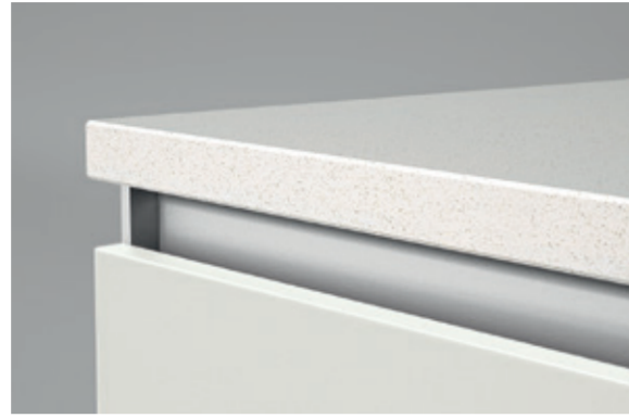
Gola in alluminio anodizzato finitura Argento Silver finish anodised Aluminium recessed grip profile . Gorge en aluminium anodisé finition Argent . Griffrielle aus eloxiertem Aluminium im Silberfinish . Gola en aluminio anodizado acabado Plata . Паз из анодированного алюминия с отделкой Серебро
