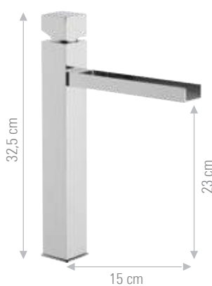
CW607B Monocomando lavabo alto con bocca a cascata, senza scarico. High basin mixer with waterfall spout, without waste.
